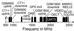
Auszug Frequenzbelegung
